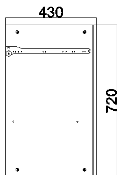
LINKE PLATTE
