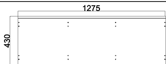
BODENPLATTE OBERSEITE
